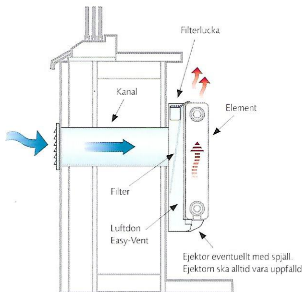
Vagg i genomskärning med kanal och luftdon Easy-Vent med monterat element
